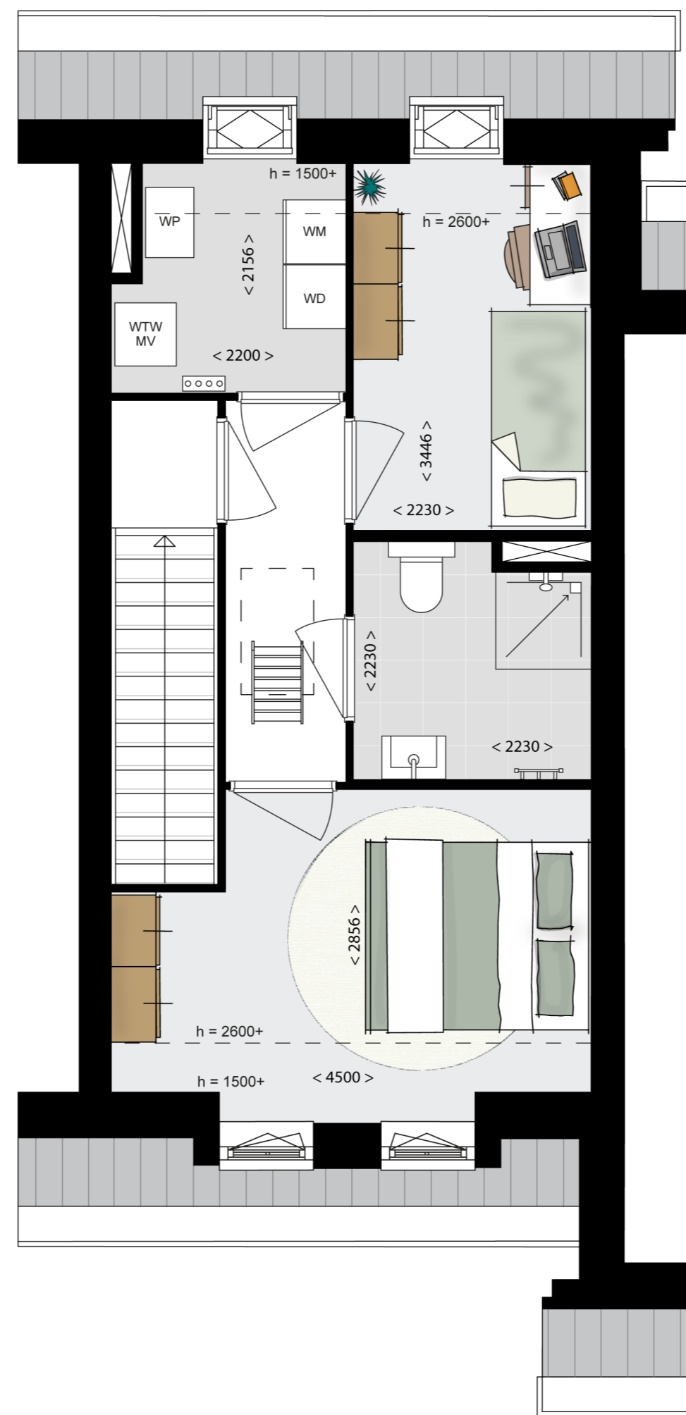
tweede verdieping
